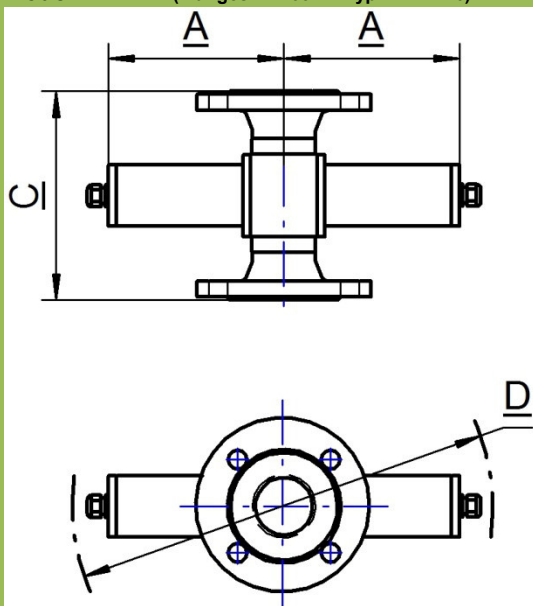
Model MTC-F (Flanges EN1092-1 Typ 11 / PN16)
